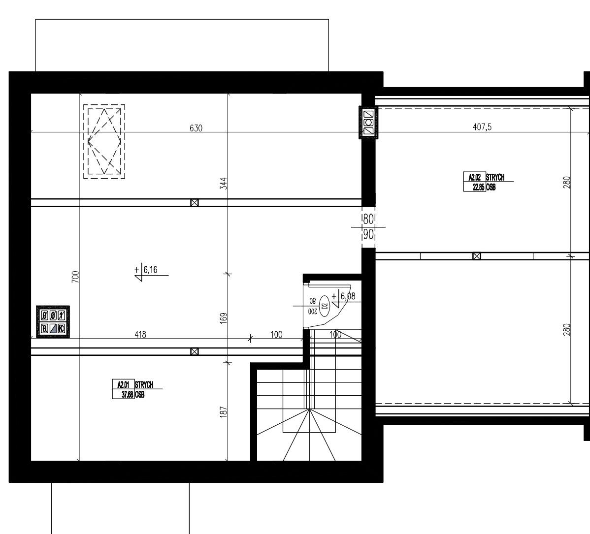
RZUT PODDASZA LOKAL A
